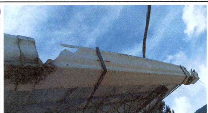
Foto 11: Cambio de canales receptores de lluvia en mal estado.
